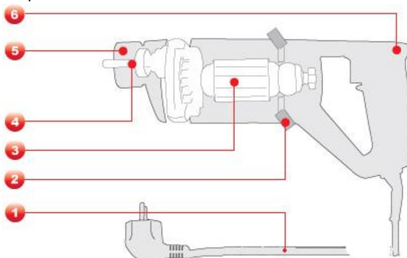
Рис.2 - Устройство электропривода
